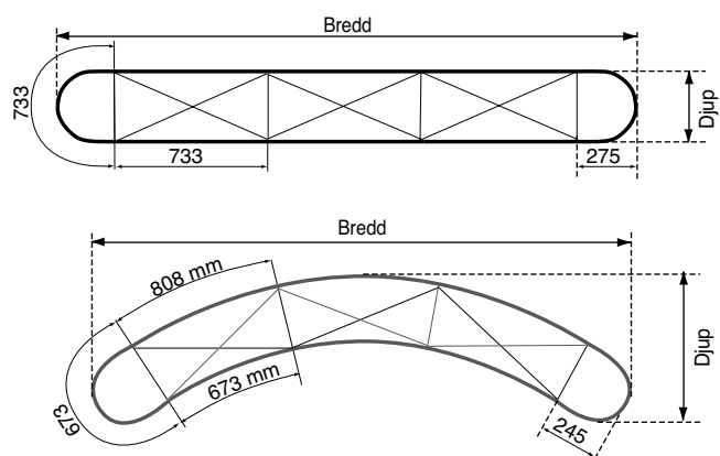
Svängda system kopplade till en cirkel
